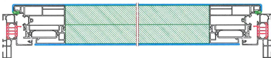
Coupe horizontale
