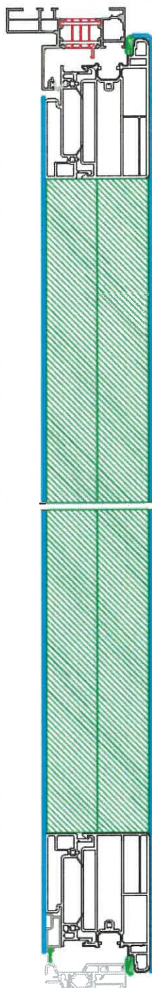
Coupe verticale
