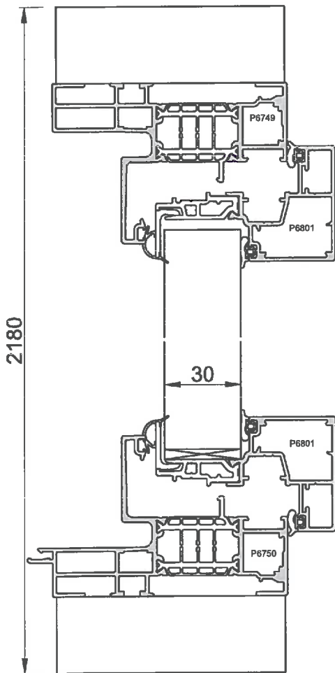
COUPE VERTICALE
