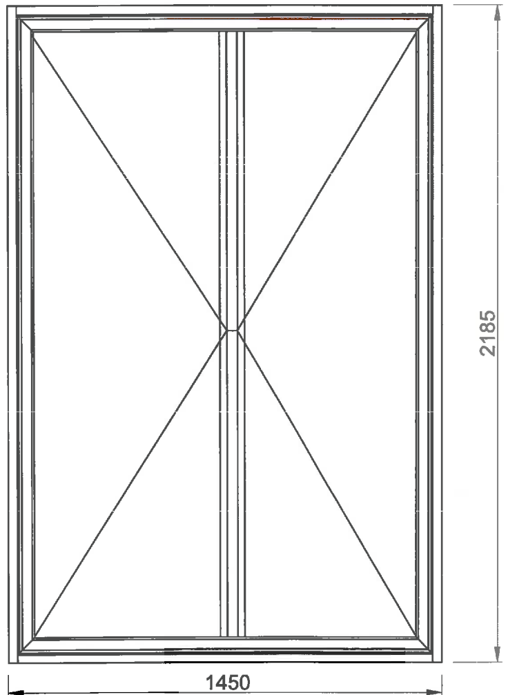
ELEVATION
