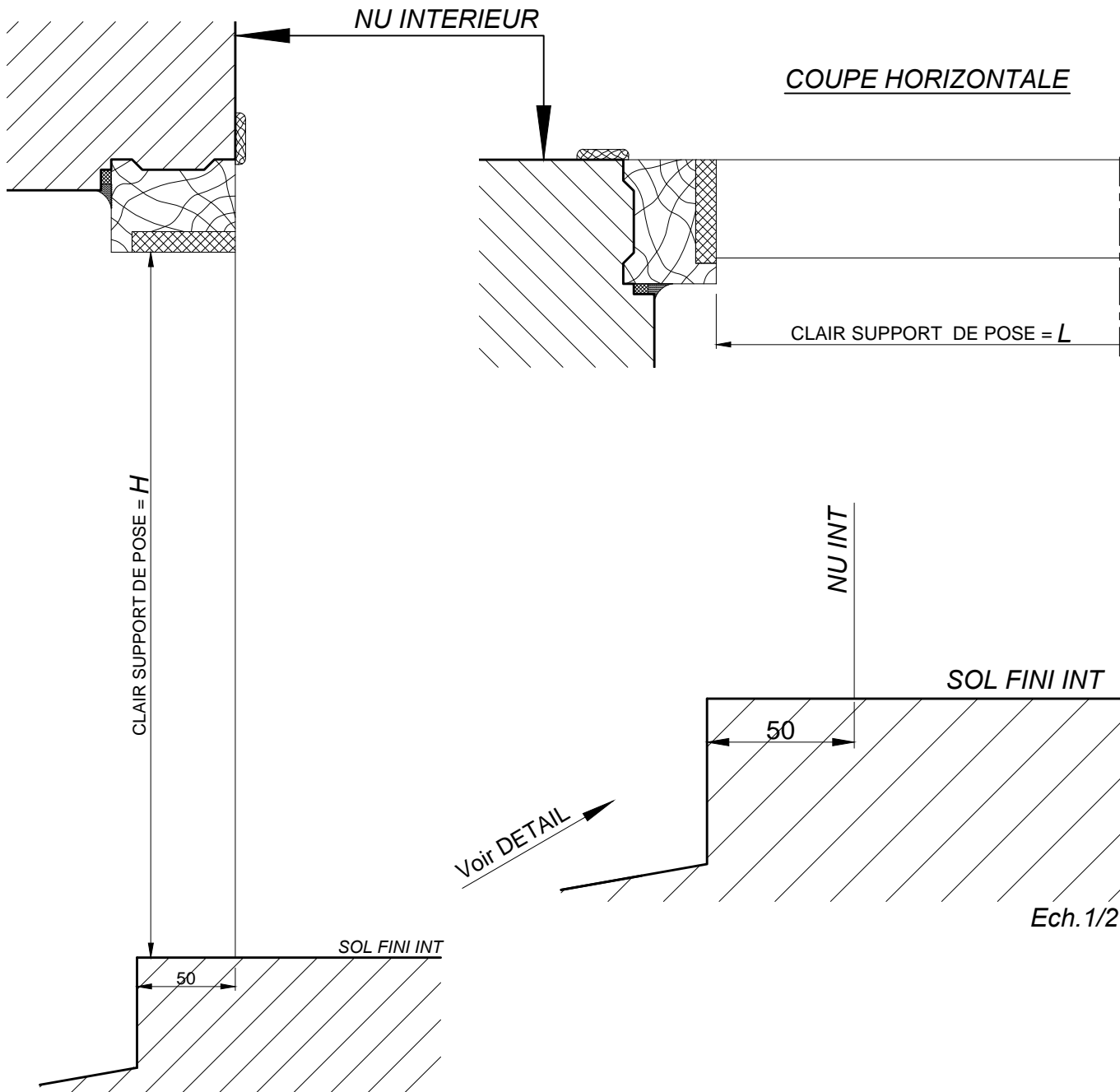
COUPE VERTICALE
