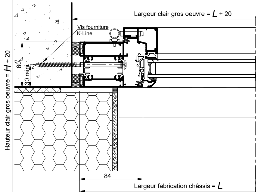
COUPE HORIZONTALE PARTIELLE Ech 1/3
