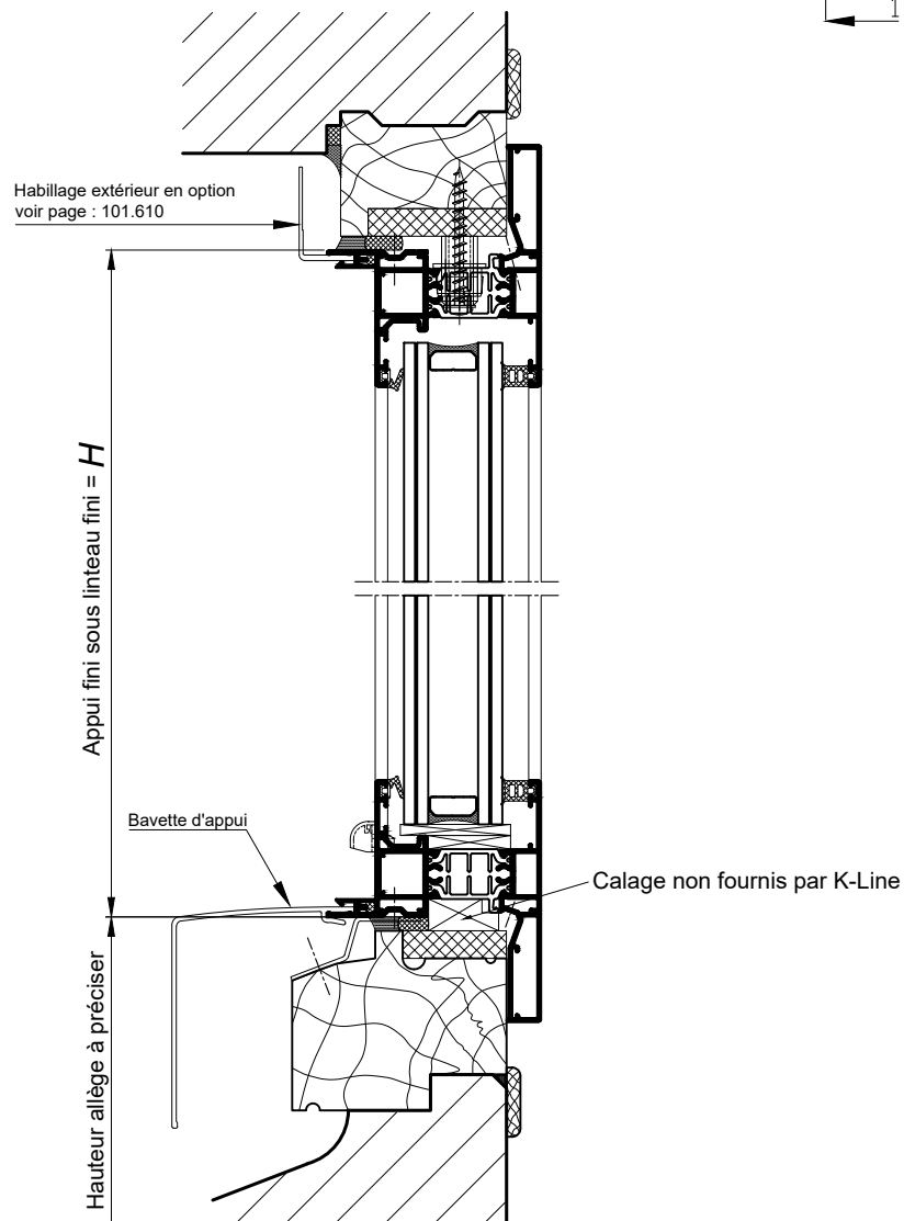
COUPE VERTICALE 1-1 Ech 1/3
