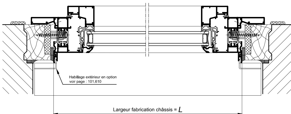
COUPE HORIZONTALE Ech 1/3
