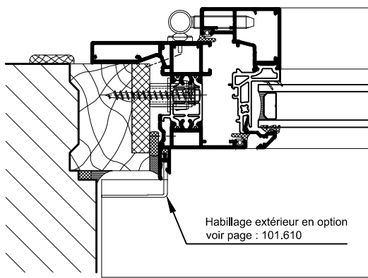
COUPE HORIZONTALE PARTIELLE Ech 1/3
