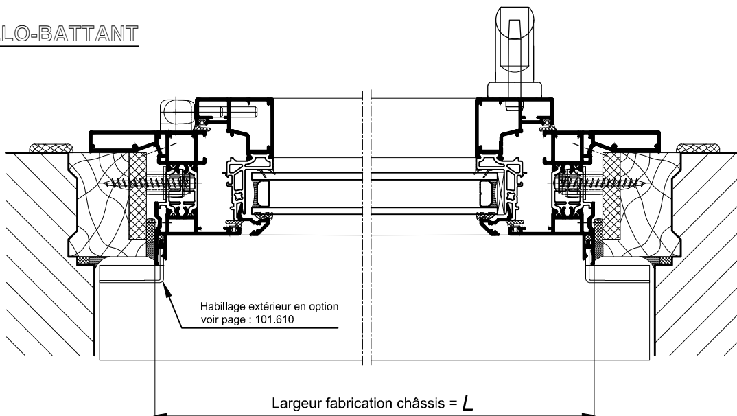
COUPE HORIZONTALE Ech 1/3
