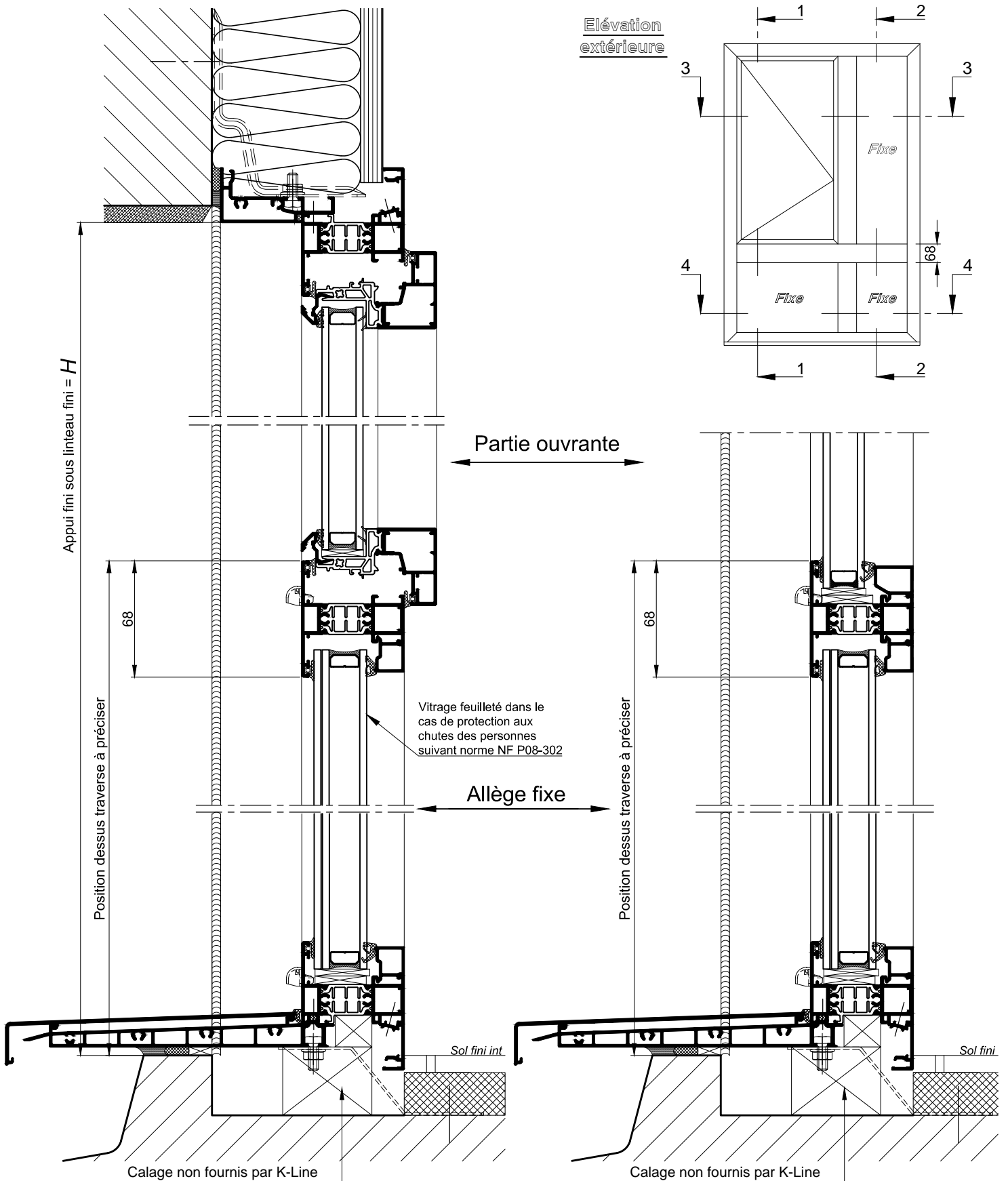
COUPE 2-2 VERTICALE PARTIELLE Ech 1/3
