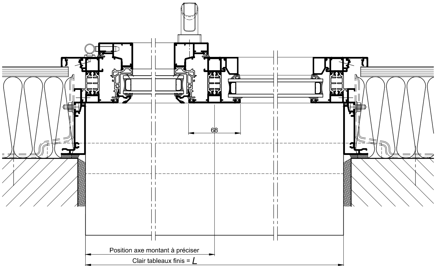
COUPE 3-3 HORIZONTALE Ech 1/3
