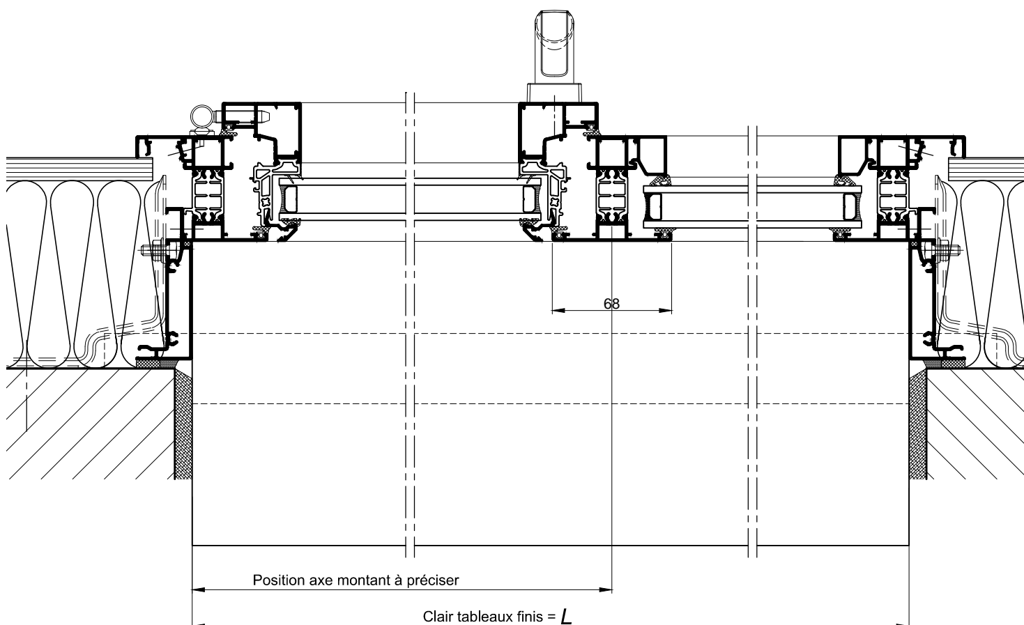
COUPE 1-1 HORIZONTALE Ech 1/3
