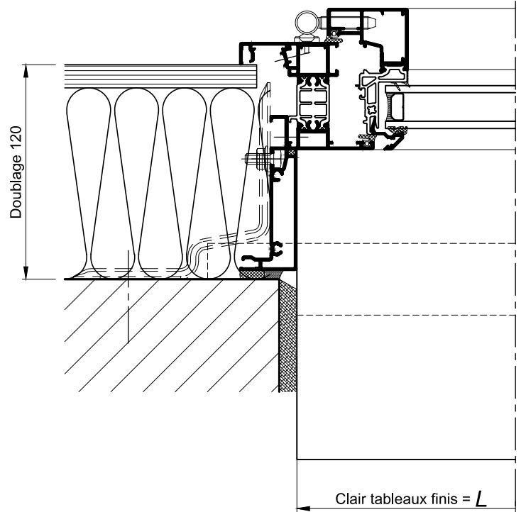
COUPE HORIZONTALE PARTIELLE Ech 1/3
