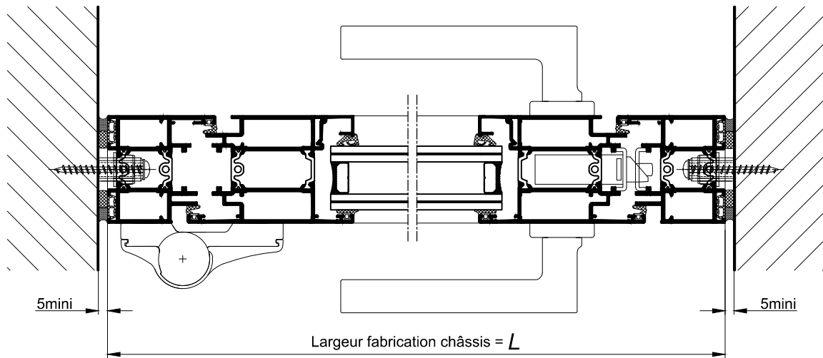
COUPE HORIZONTALE 2-2 Ech 1/3
