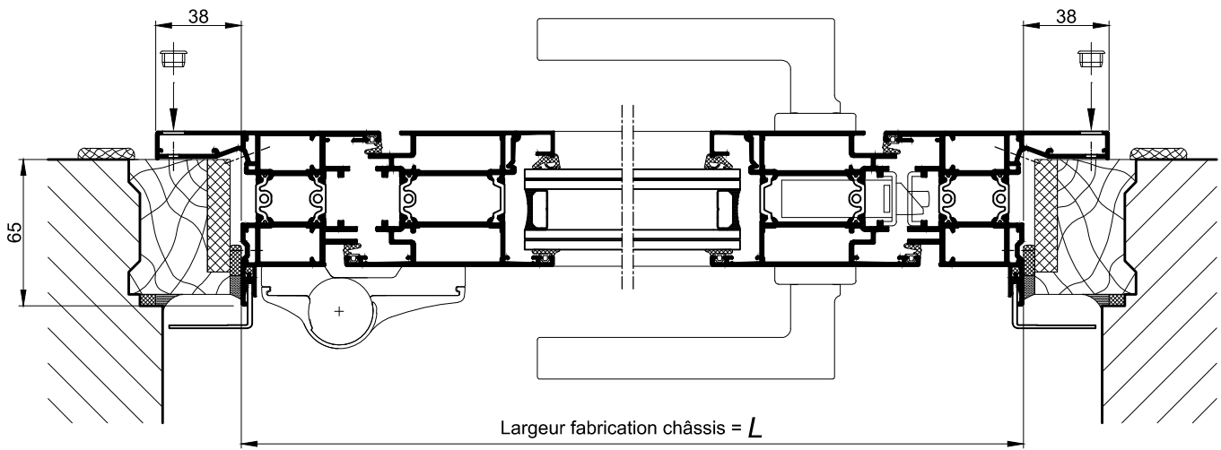
COUPE HORIZONTALE 2-2 Ech 1/3
