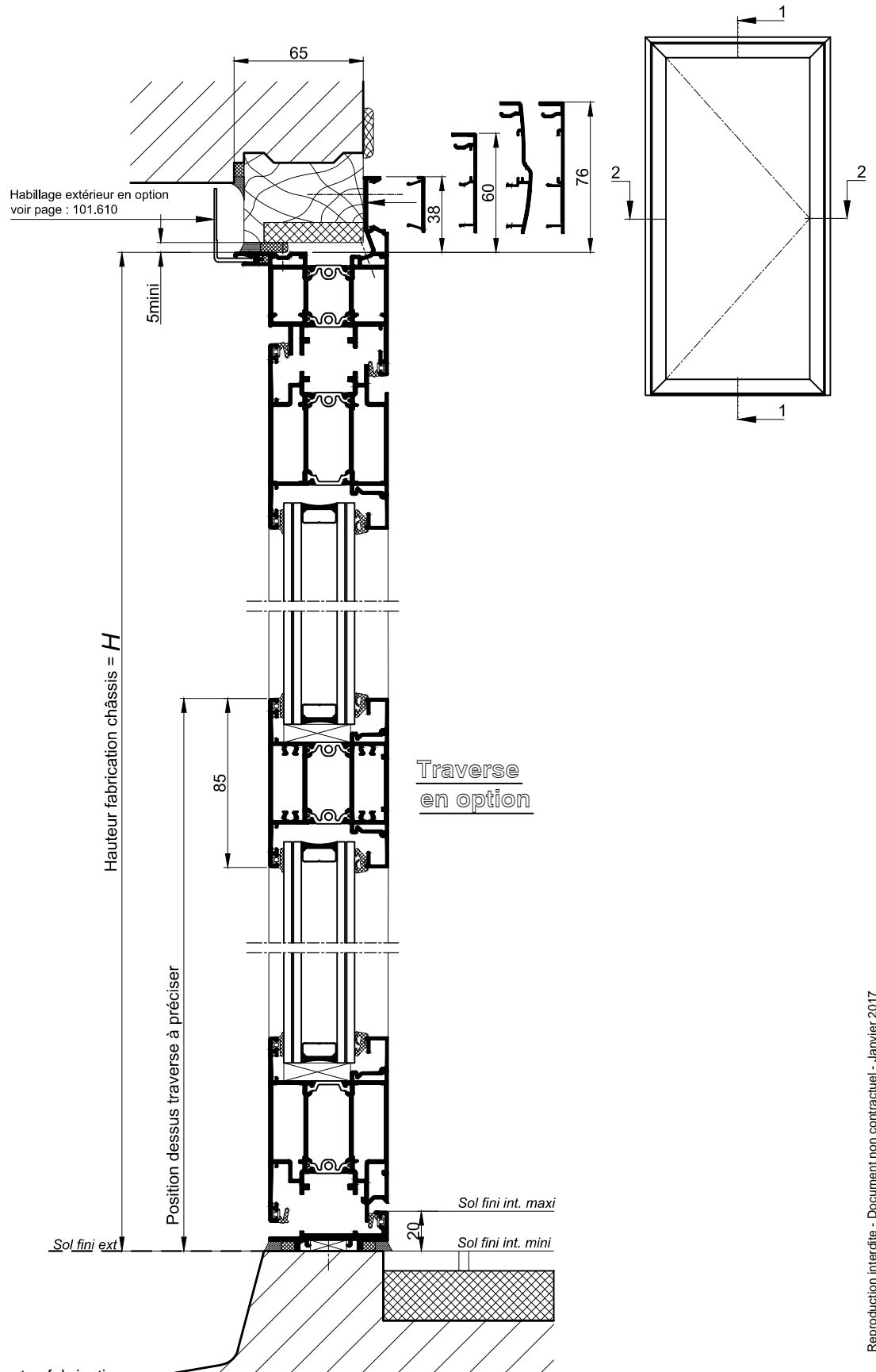
COUPE VERTICALE 1-1 Ech 1/3
