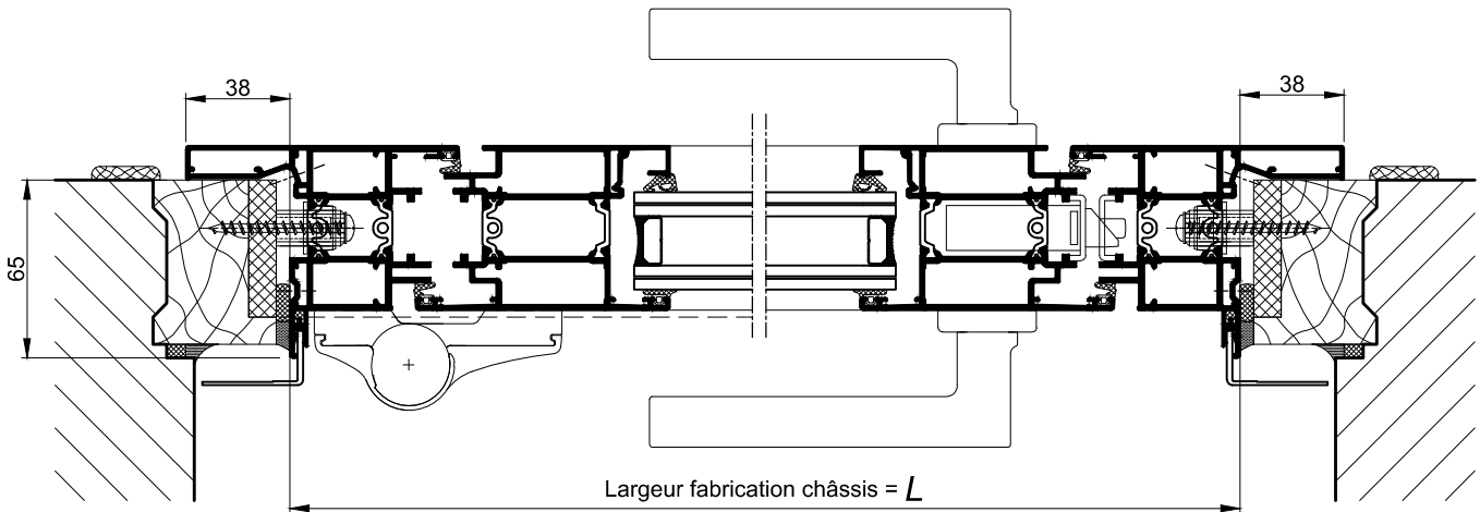
COUPE HORIZONTALE 2-2 Ech 1/3
