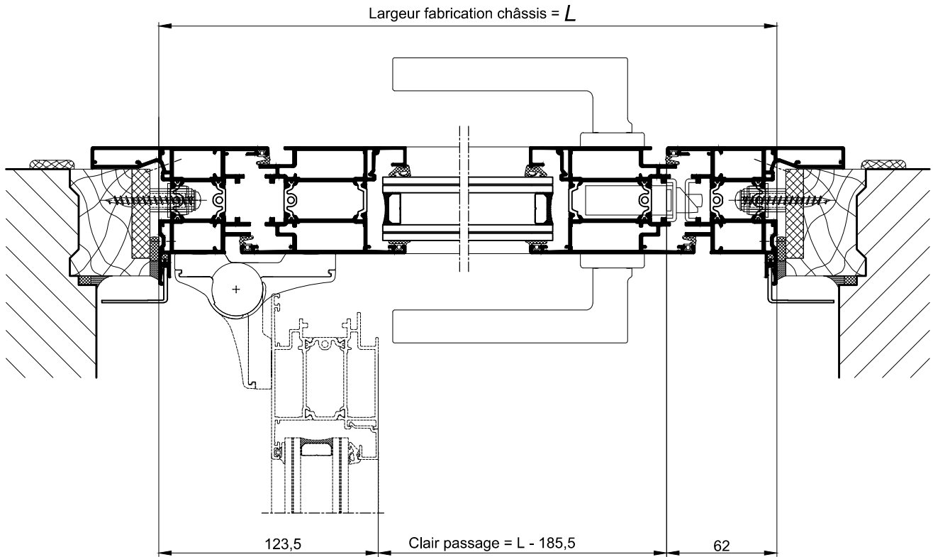
COUPE HORIZONTALE 2-2 Ech 1/3
