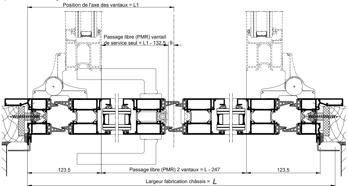
COUPE HORIZONTALE 3-3
