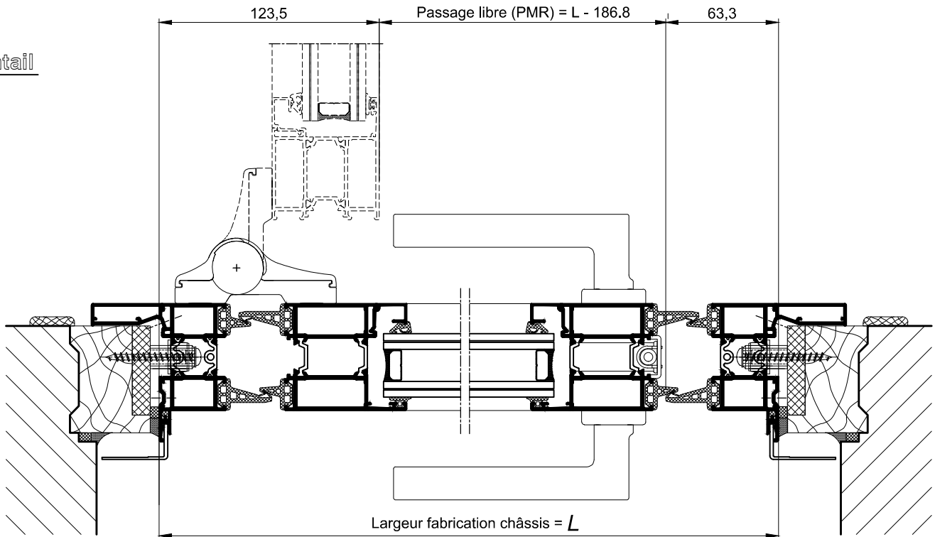
COUPE HORIZONTALE 2-2
