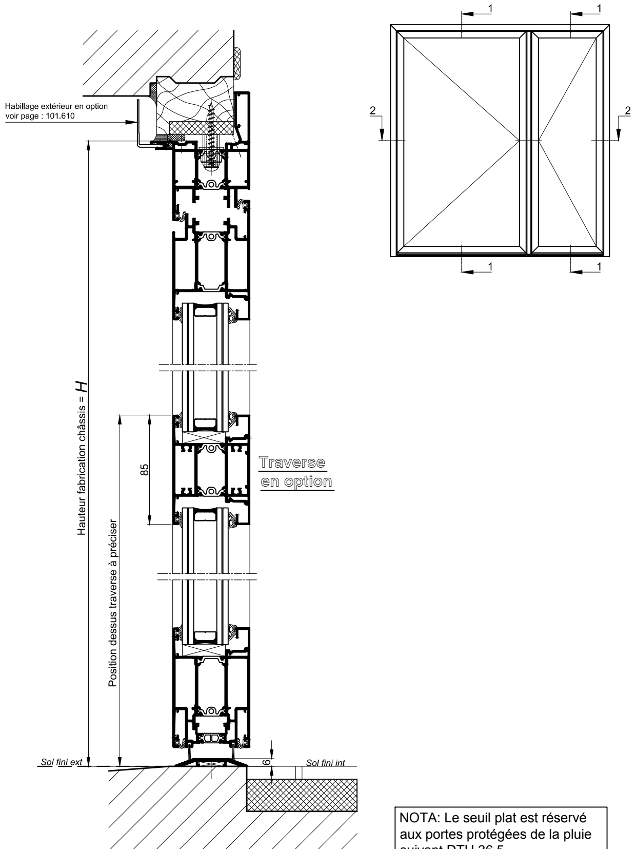
COUPE VERTICALE Ech 1-1 1/3
