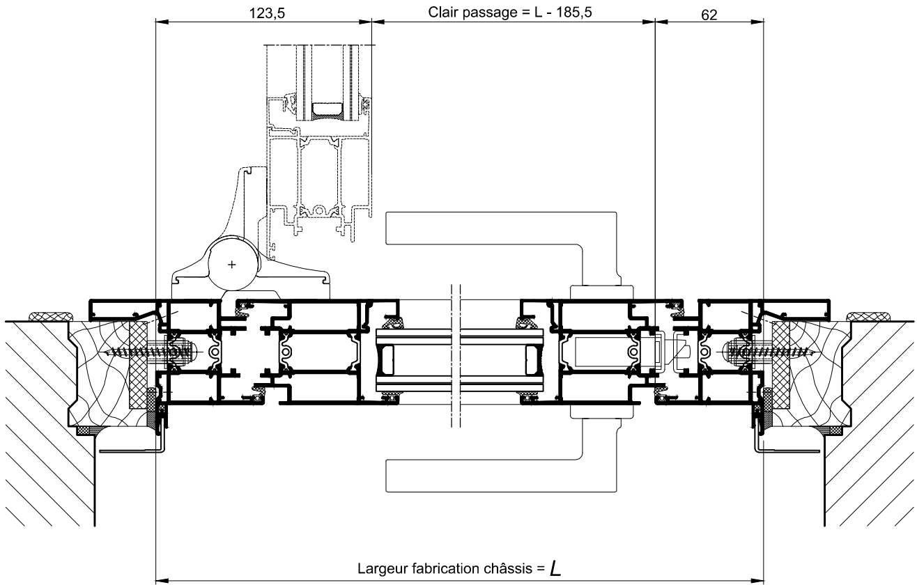
COUPE HORIZONTALE 2-2 Ech 1/3
