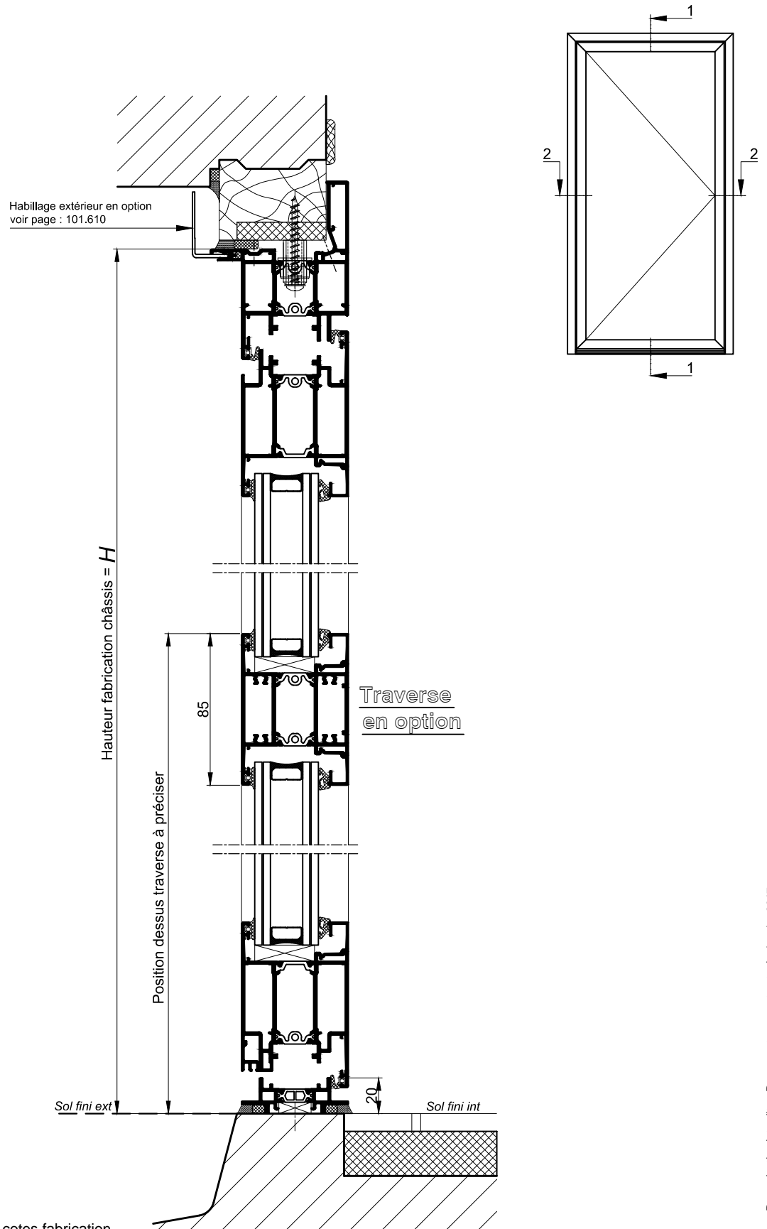
COUPE VERTICALE 1-1 Ech 1/3
