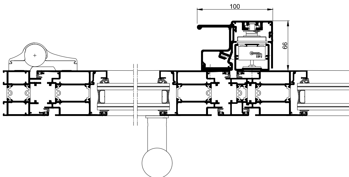
COUPE HORIZONTALE 3-3 Ech 1/3
