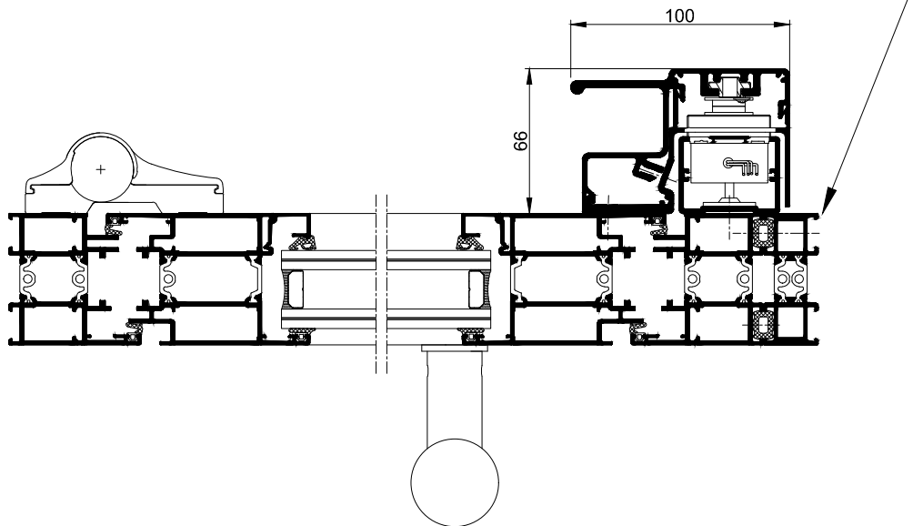
COUPE HORIZONTALE 2-2 Ech 1/3
