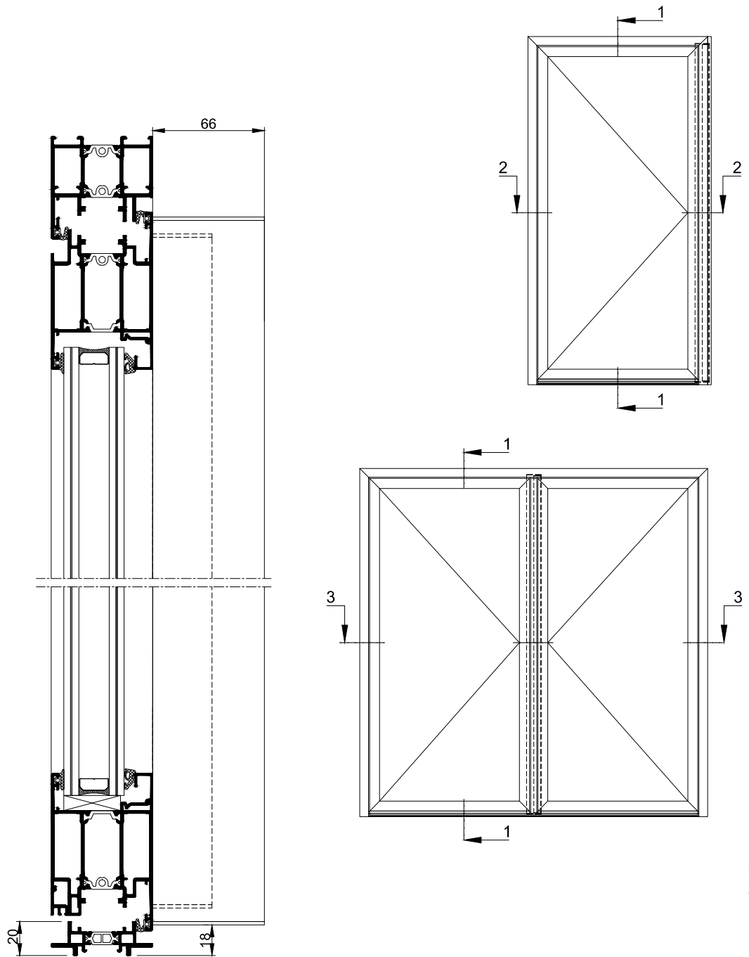
COUPE VERTICALE 1-1 Ech 1/3
