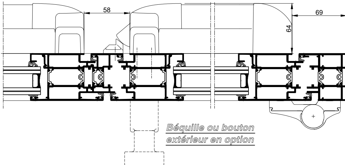
COUPE HORIZONTALE 3-3 Ech 1/3
