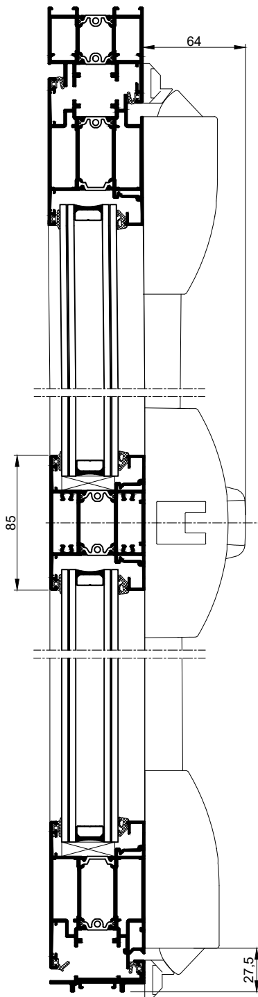
COUPE VERTICALE 1-1 Ech1/3
