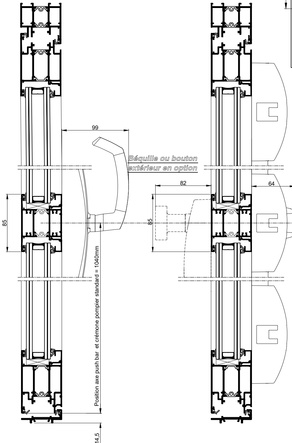
COUPE VERTICALE 1-1 Ech1/3
