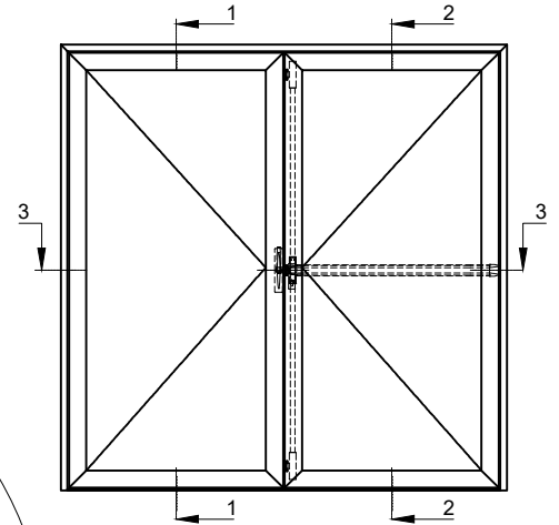
Vantail de service
