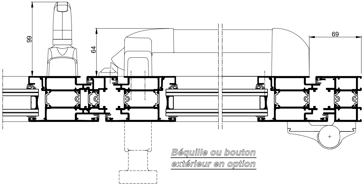
COUPE HORIZONTALE 3-3 Ech 1/3
