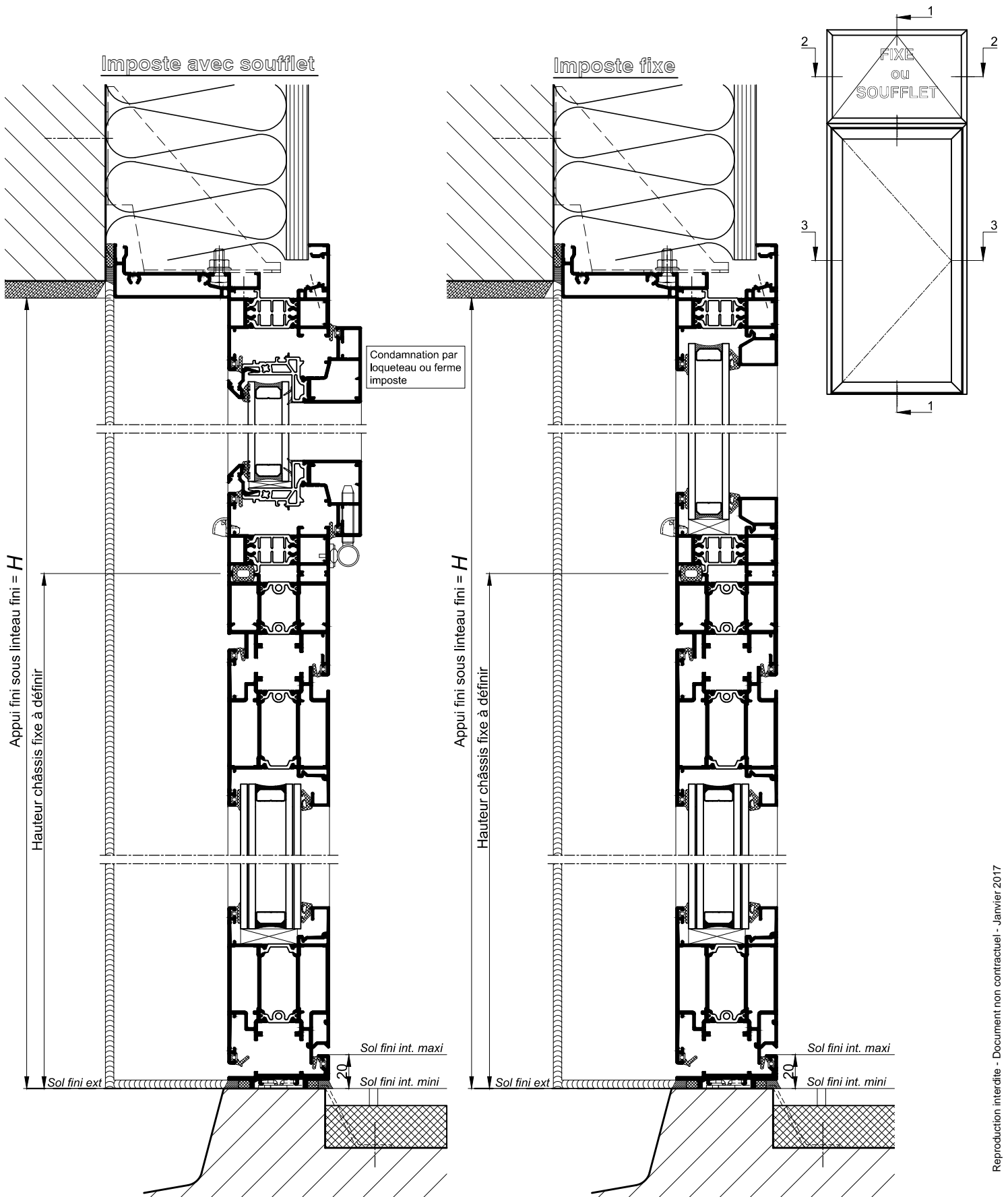
COUPES VERTICALES 1-1
