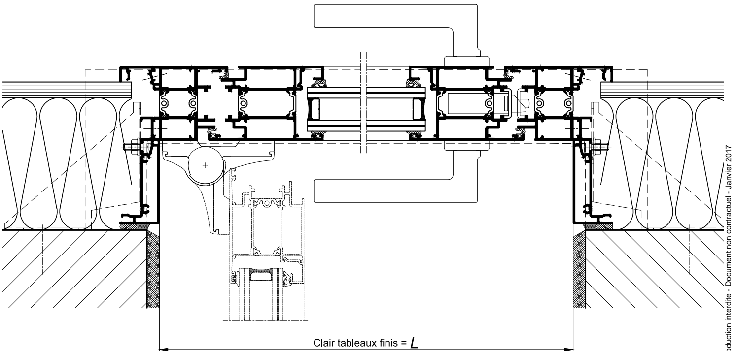
COUPE HORIZONTALE 3-3 Ech 1/3
