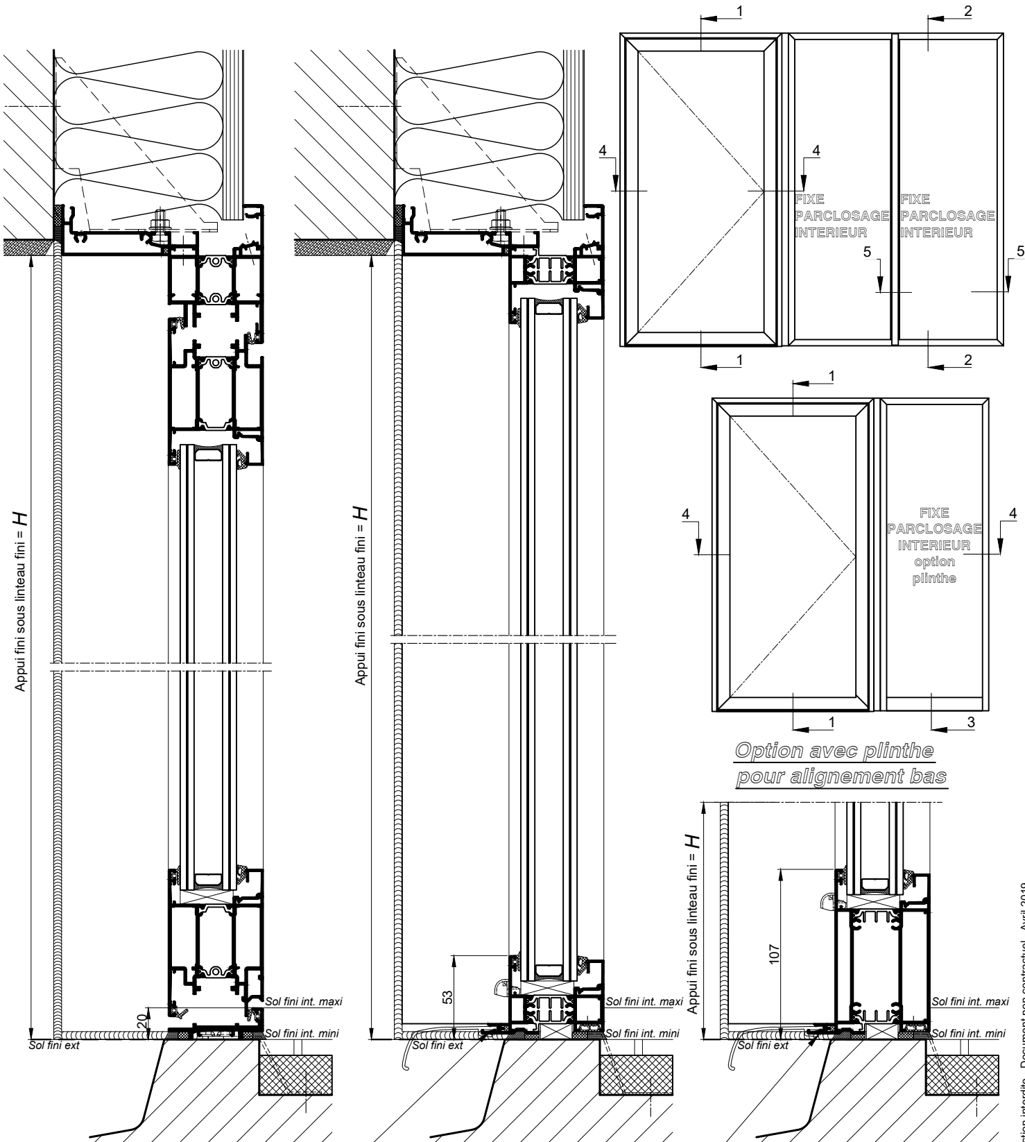
COUPE VERTICALE 1-1 Ech 1/3
