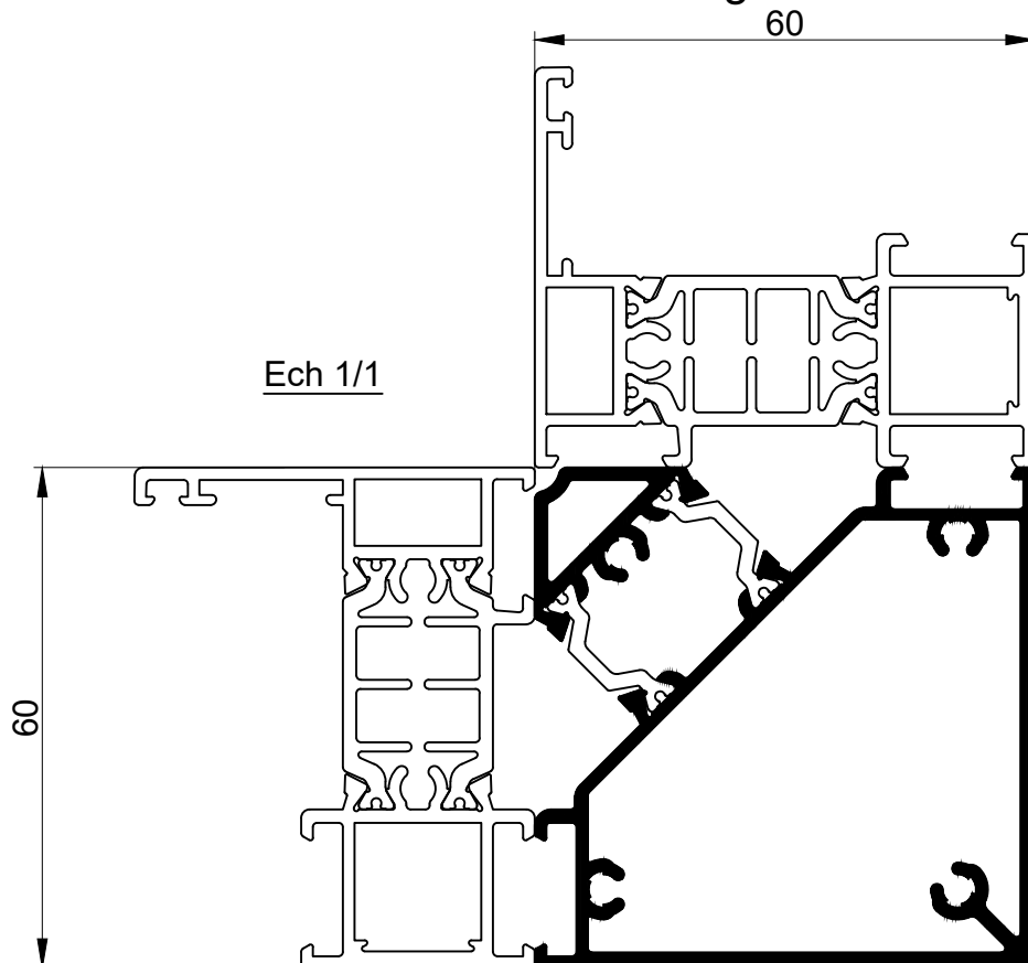
Profil d'angle 90°
