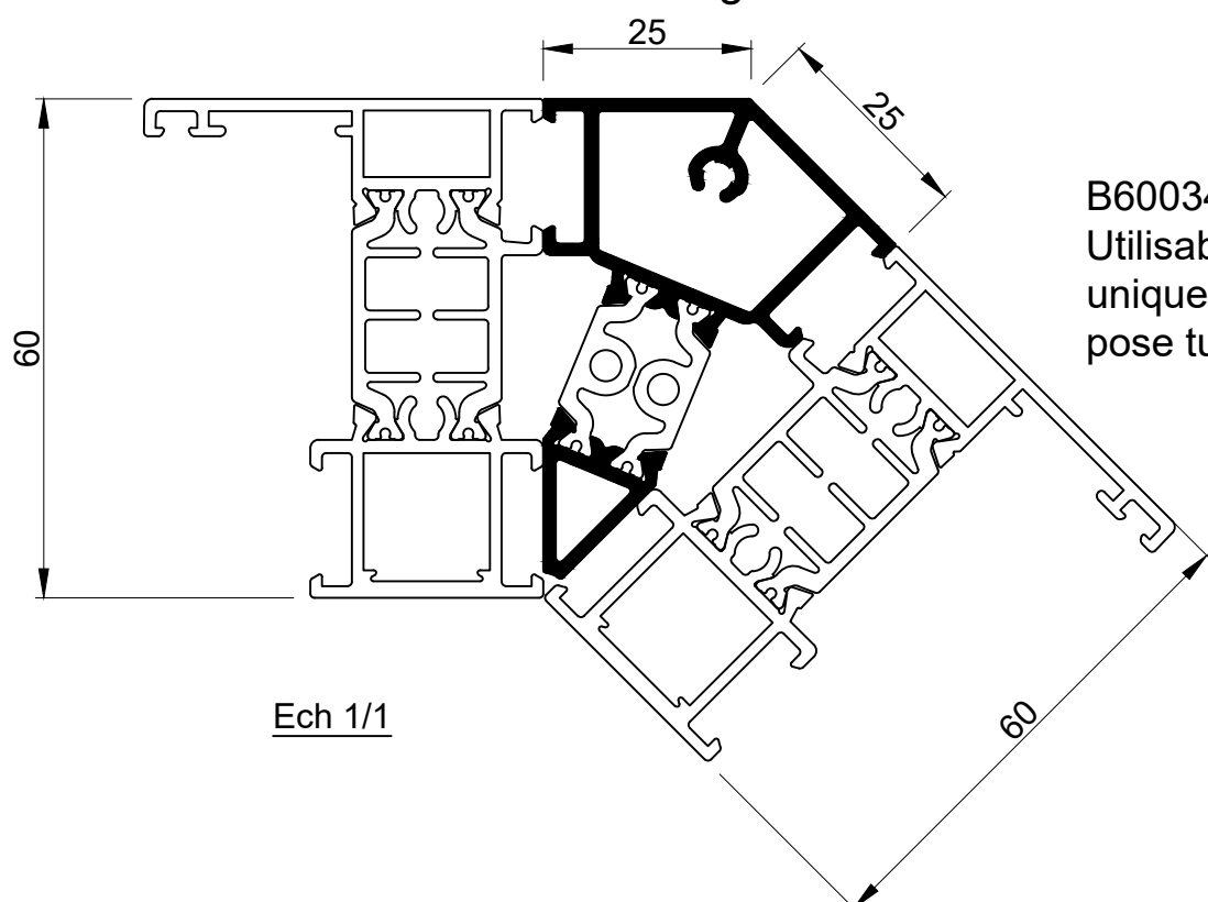
Profil d'angle 135°
