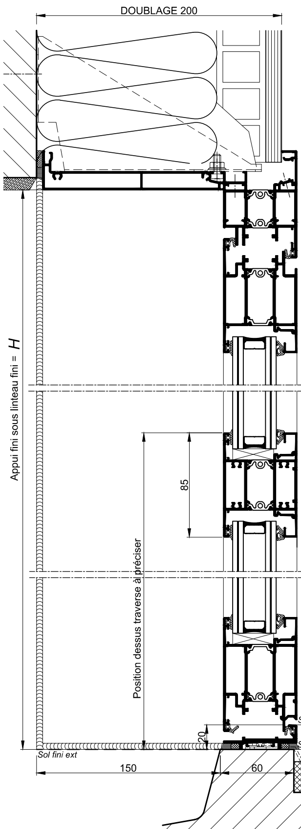
COUPE VERTICALE 1-1 Ech 1/3
