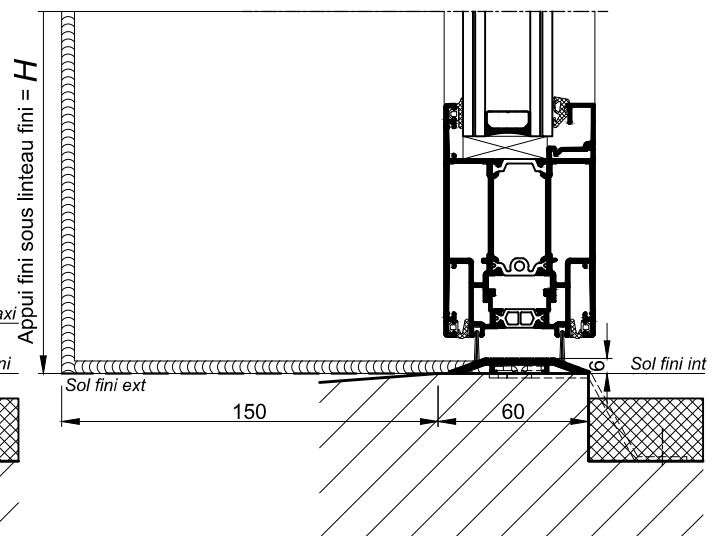
COUPE VERTICALE PARTIELLE 1-1 Ech 1/3
