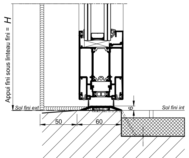
COUPE VERTICALE PARTIELLE 1-1 Ech 1/3
