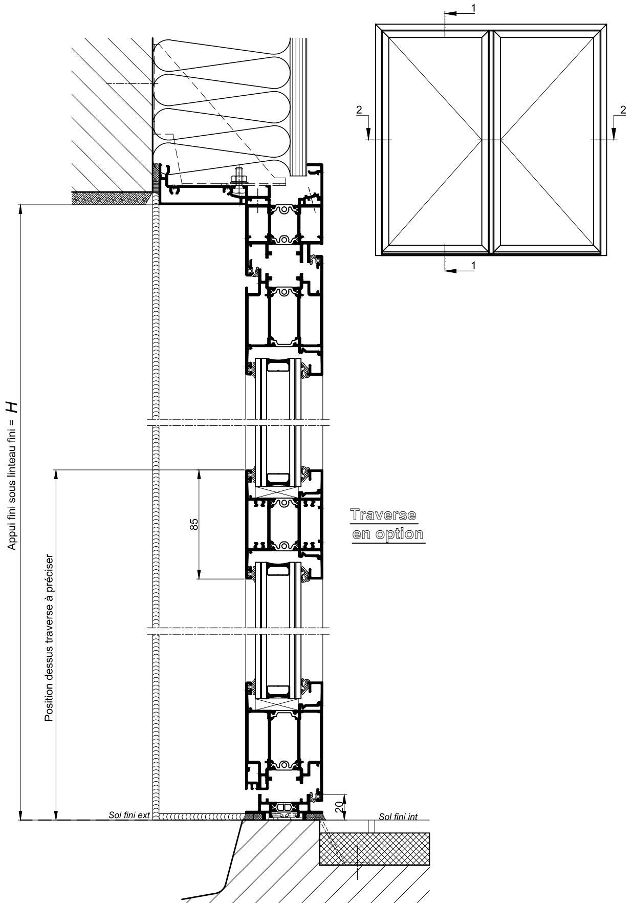
COUPE VERTICALE 1-1
