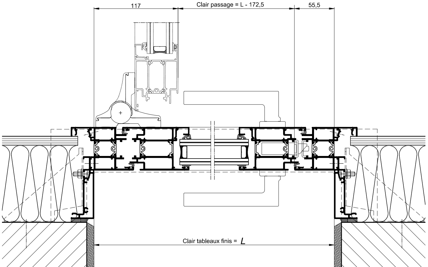
COUPE HORIZONTALE 2-2
