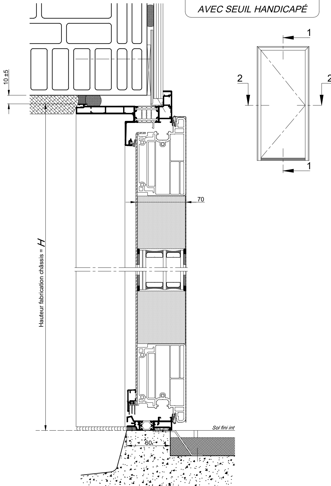
COUPE 1-1 VERTICALE Ech 1/3
