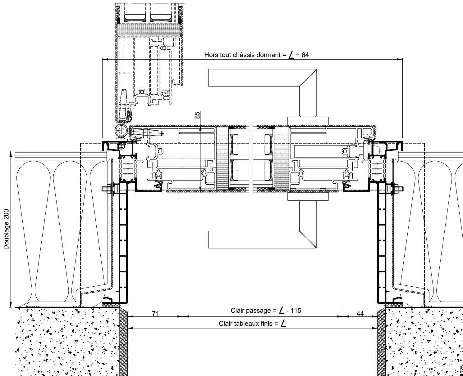
COUPE 2-2 HORIZONTALE Ech 1/3
