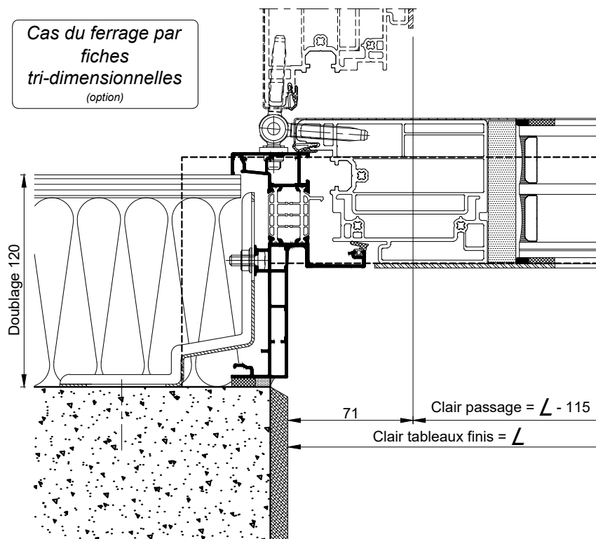
COUPE 2-2 HORIZONTALE Ech 1/3
