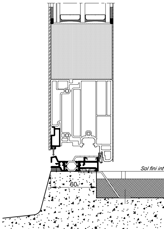
COUPE 1-1 VERTICALE Ech 1/3
