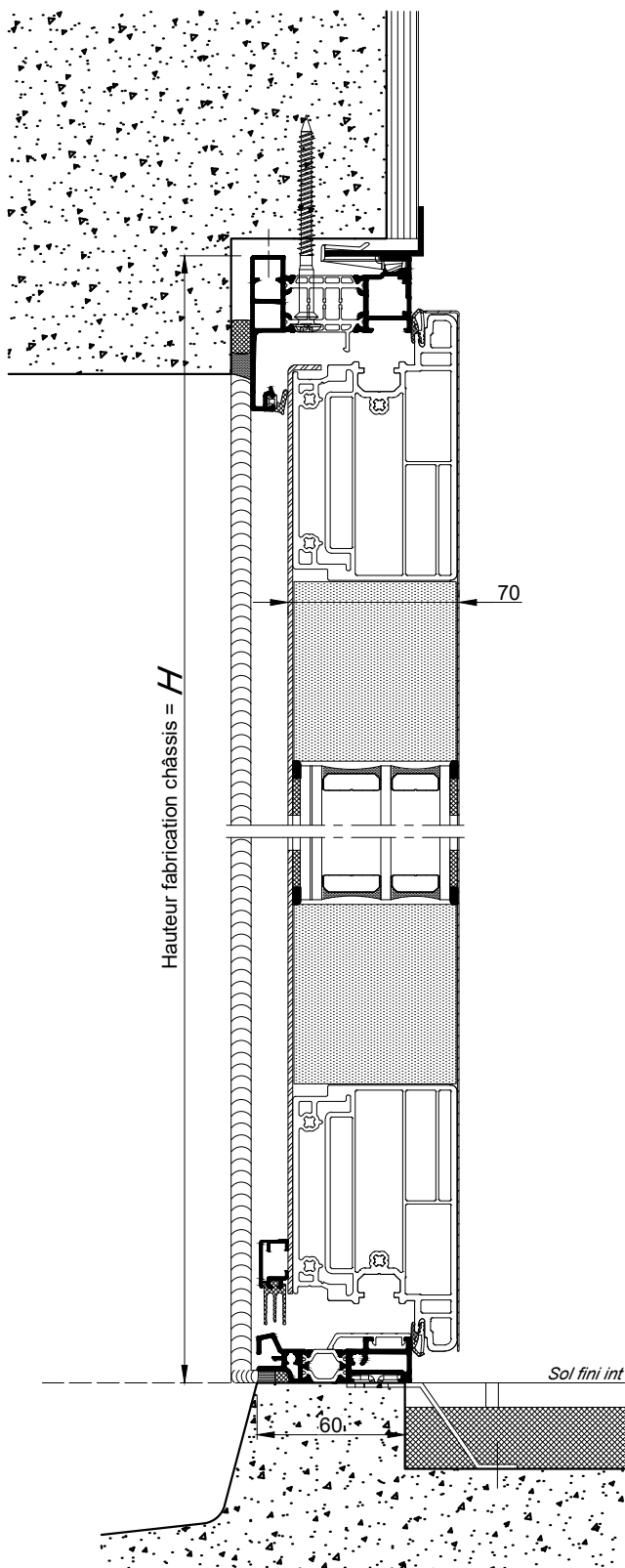
COUPE 1-1 VERTICALE Ech 1/3
