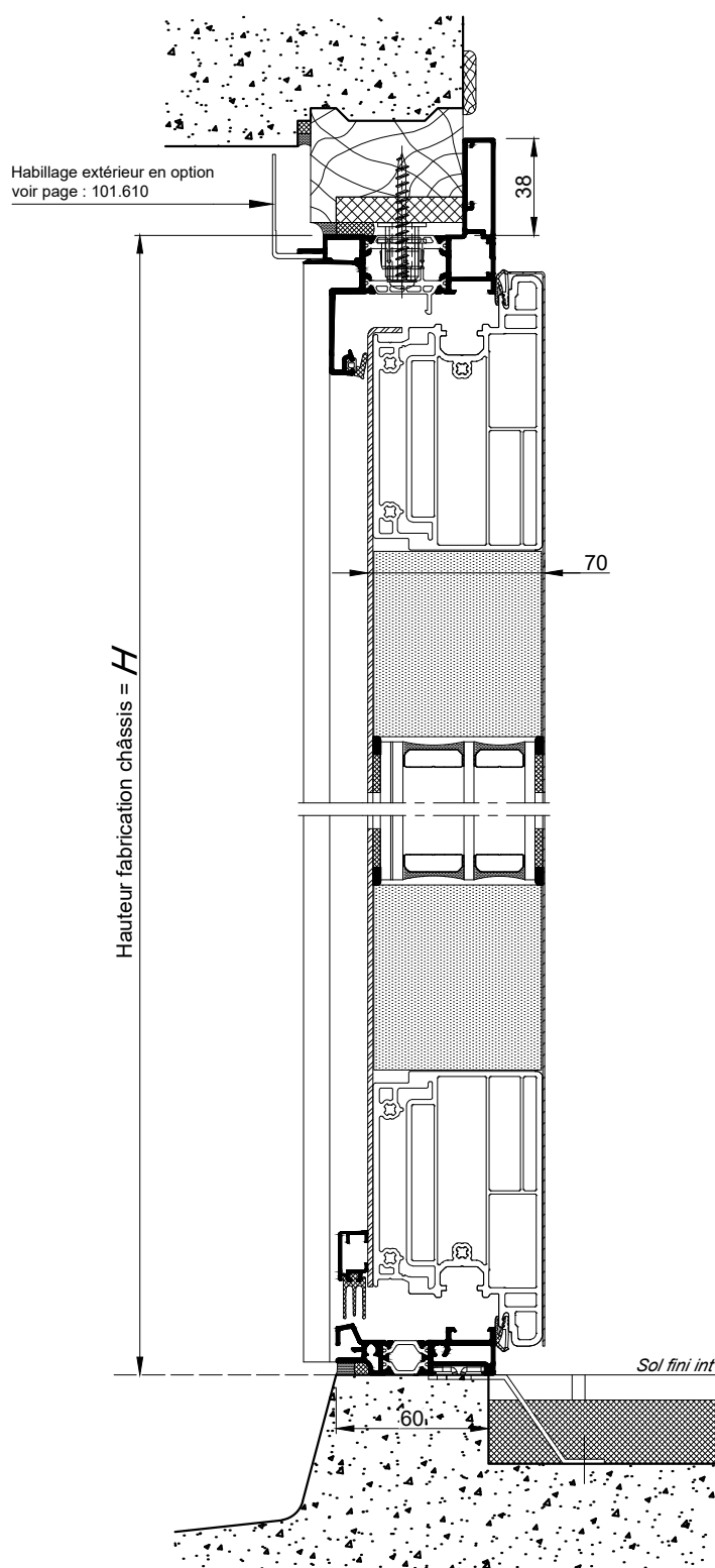
COUPE 1-1 VERTICALE Ech 1/3
