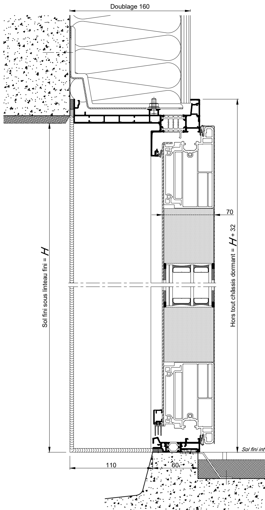
COUPE 1-1 VERTICALE Ech 1/3
