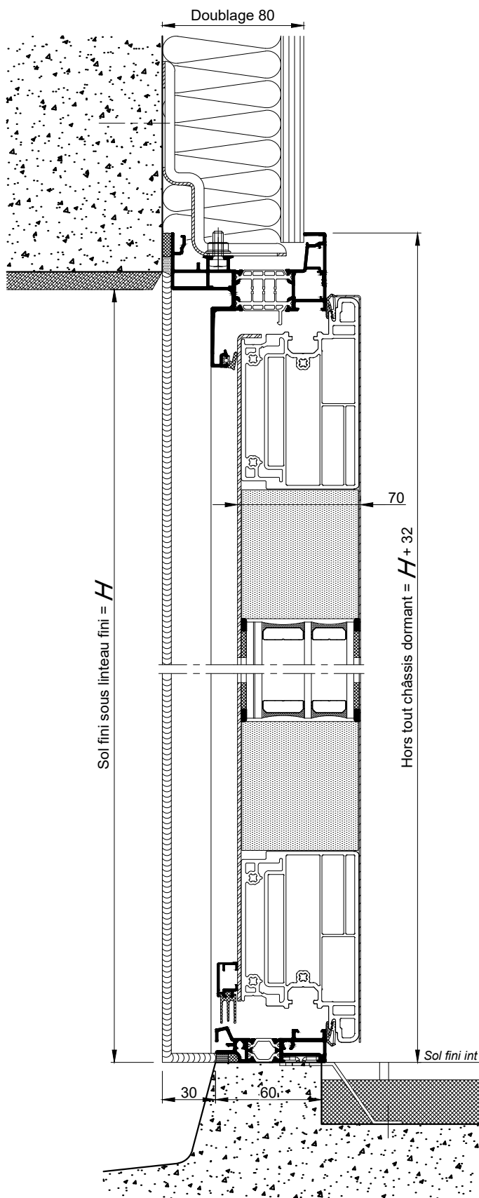
COUPE 1-1 VERTICALE Ech 1/3
