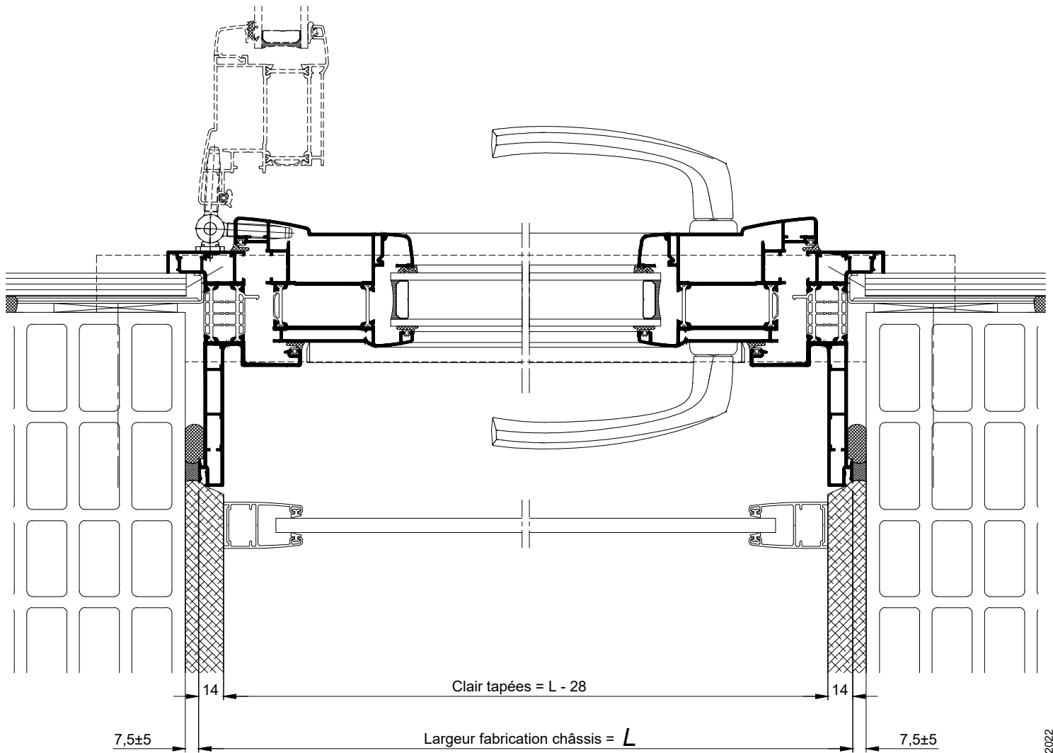
COUPE HORIZONTALE Ech 1/3
