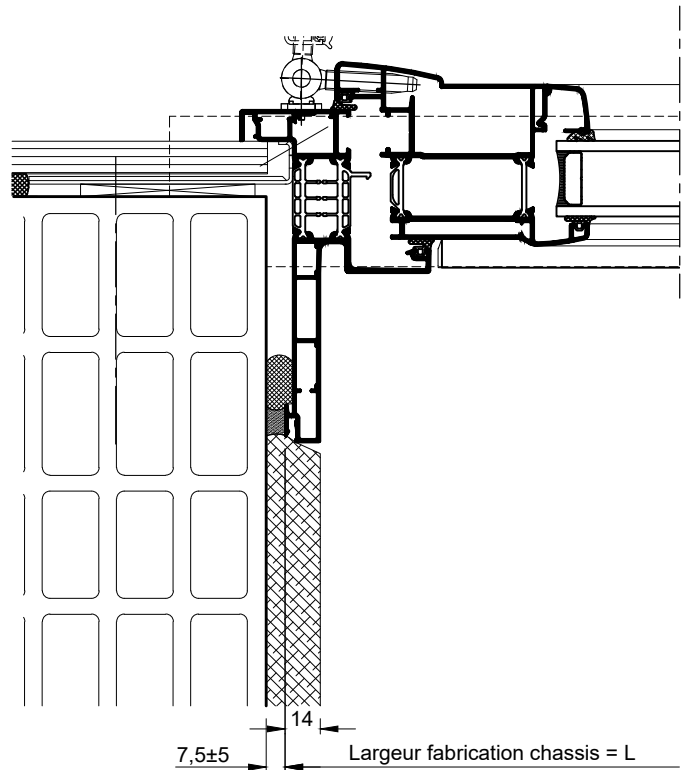
COUPE HORIZONTALE Ech 1/3
