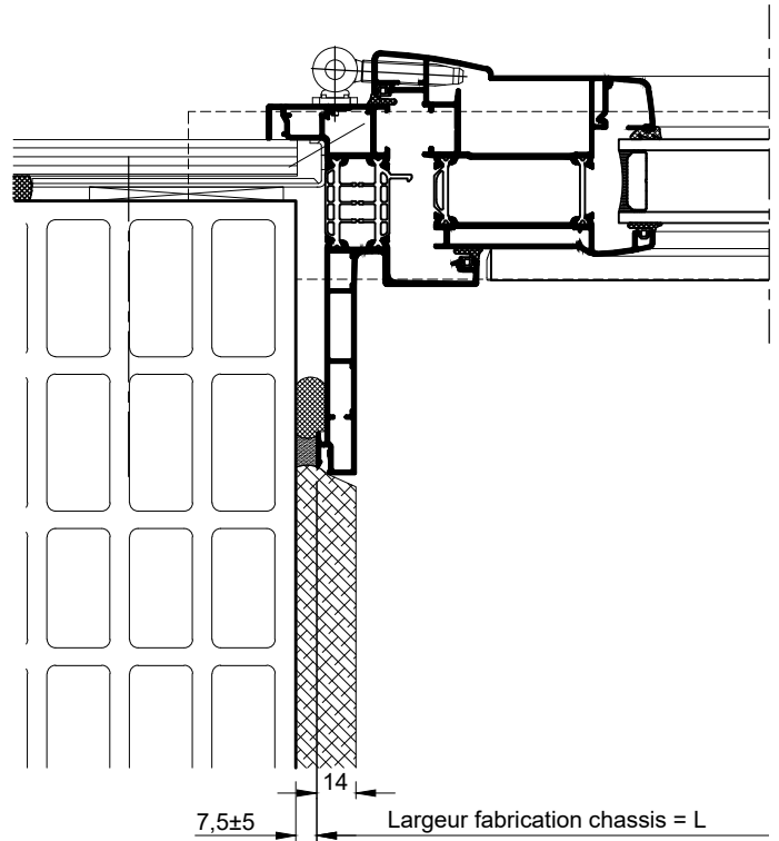
COUPE HORIZONTALE Ech 1/3
