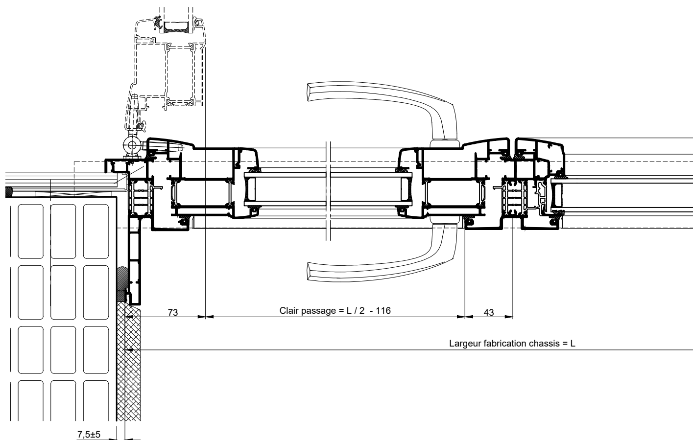
COUPE HORIZONTALE PARTIELLE Ech 1/3
