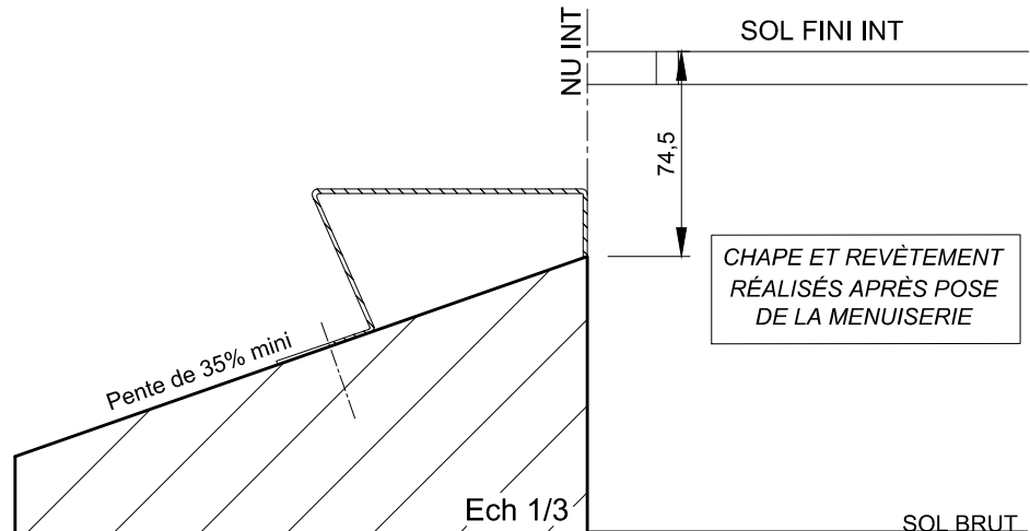
DETAIL : ENCASTREMENT DE 50 MM (VALABLE ÉGALEMENT POUR PASSAGE HANDICAPÉ)
