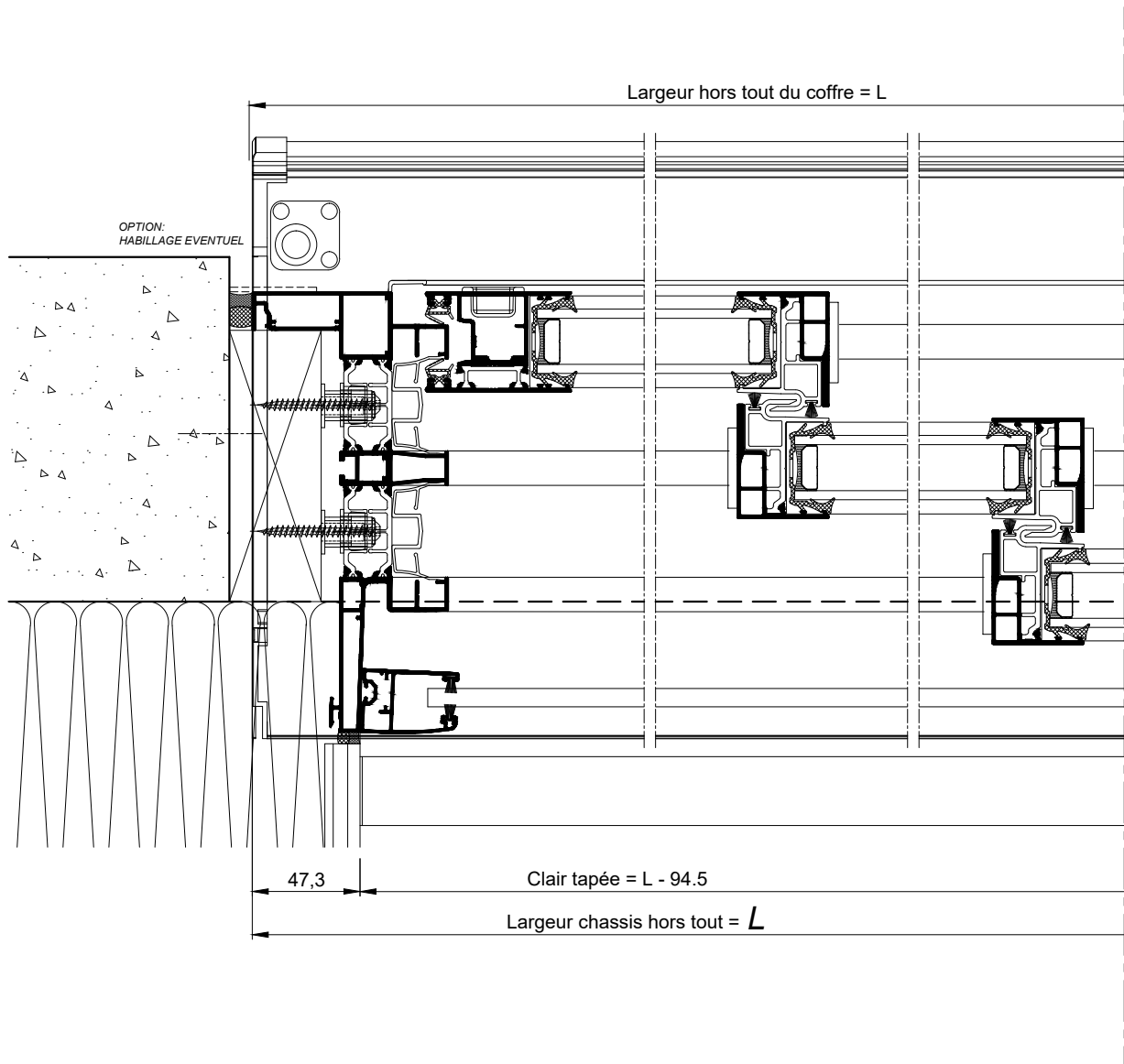
COUPE HORIZONTALE Ech 1/3
