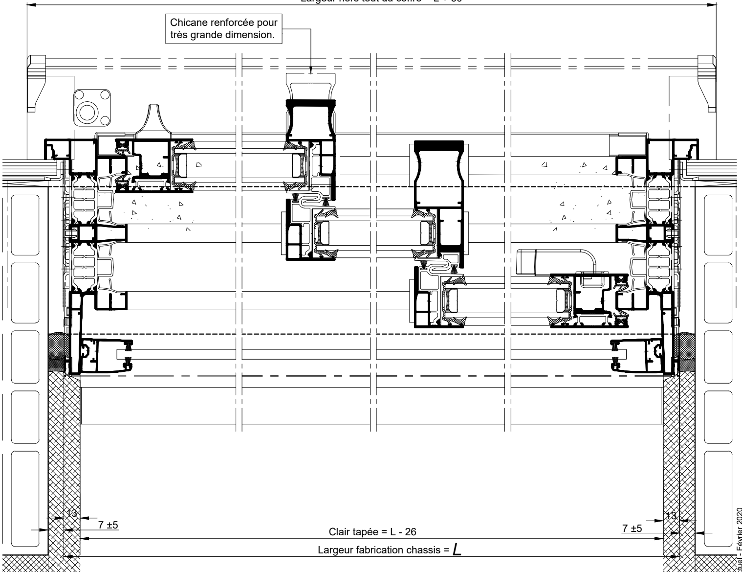
COUPE HORIZONTALE Ech 1/3
