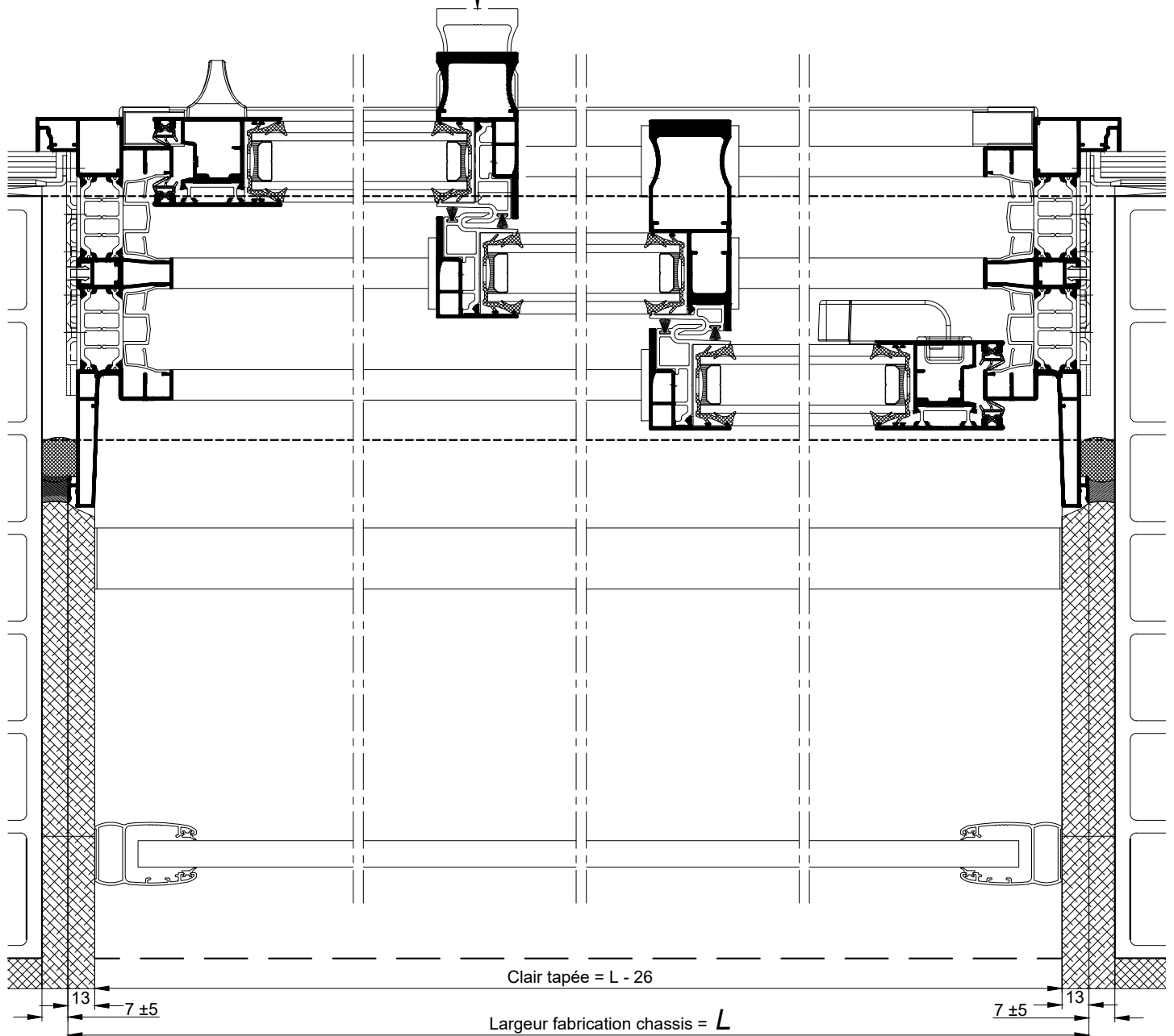
COUPE HORIZONTALE Ech 1/3
