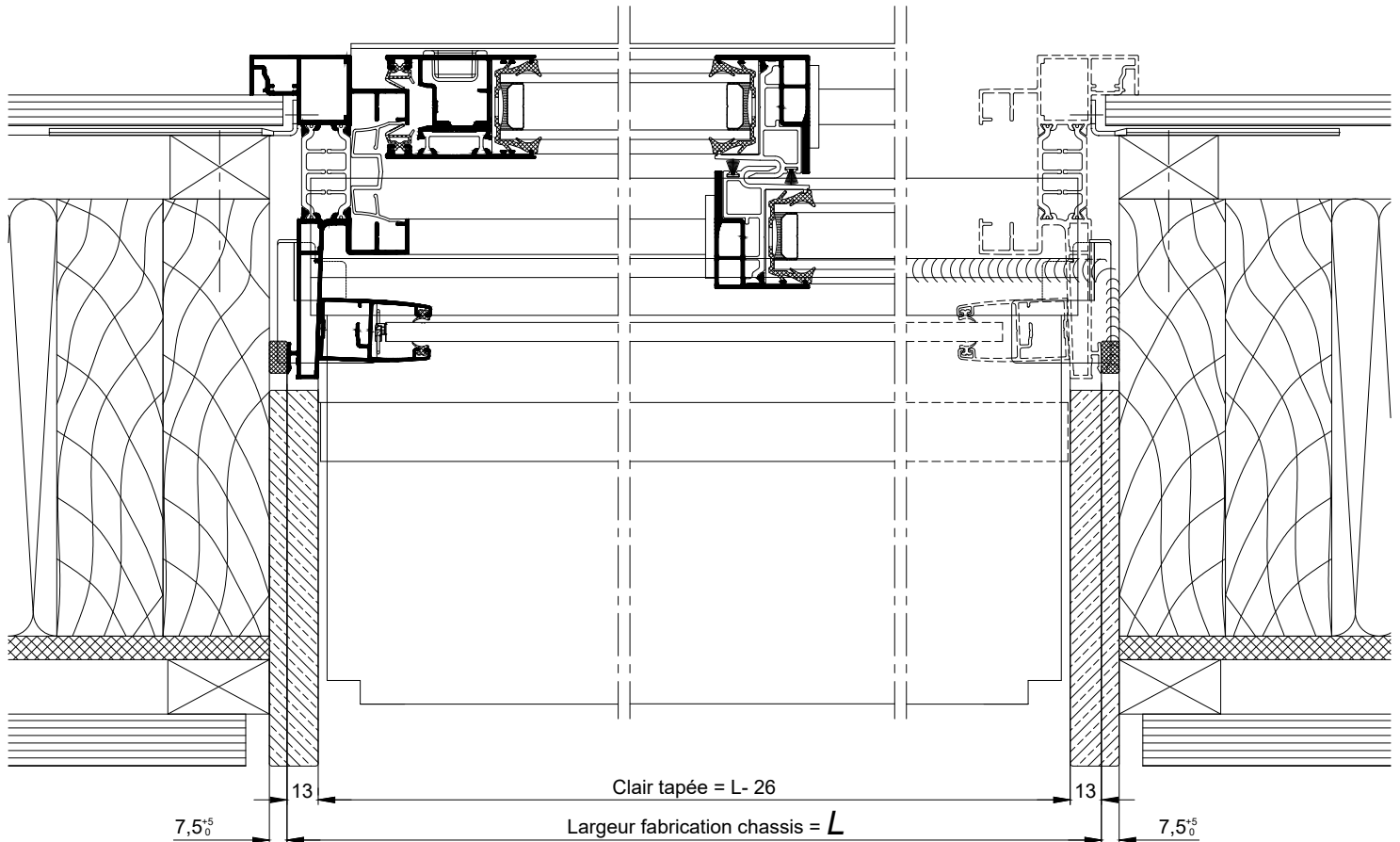
COUPE AU DROIT DE LA MENUISERIE
