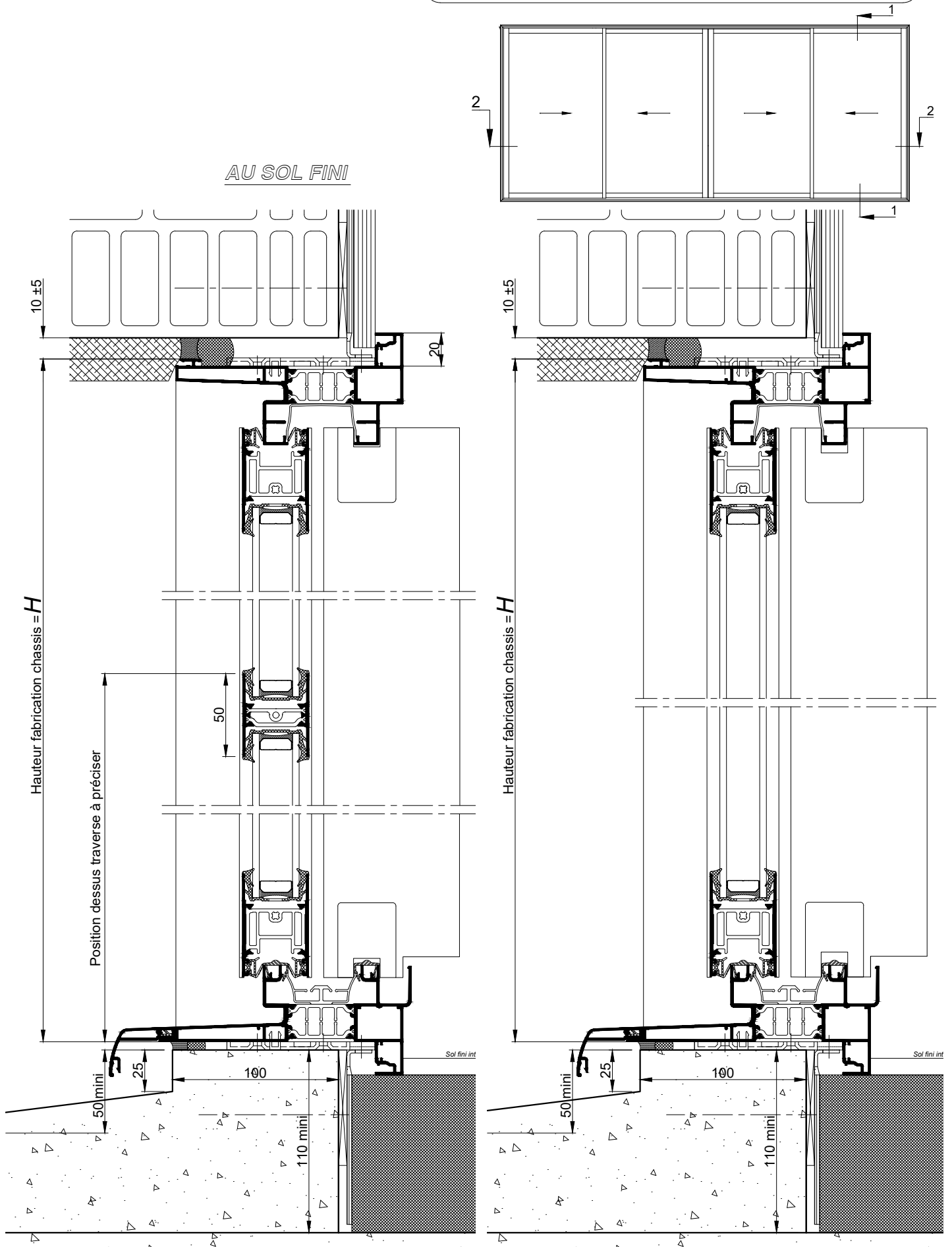
COUPES 1-1 VERTICALES Ech 1/3
