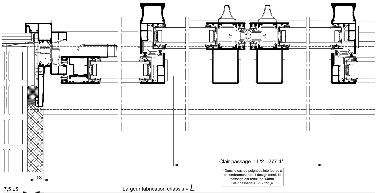
COUPES 2-2 HORIZONTALES Ech 1/3
