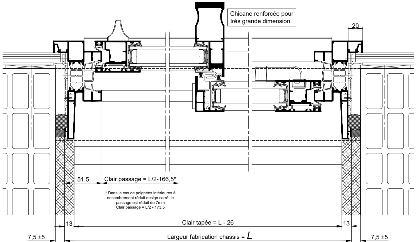
COUPES 2-2 HORIZONTALES Ech 1/3
