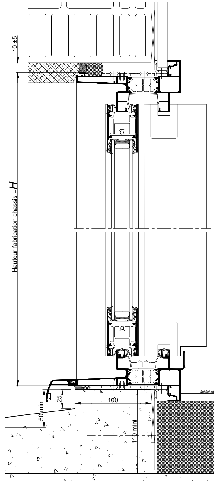
COUPES 1-1 VERTICALES Ech 1/3
