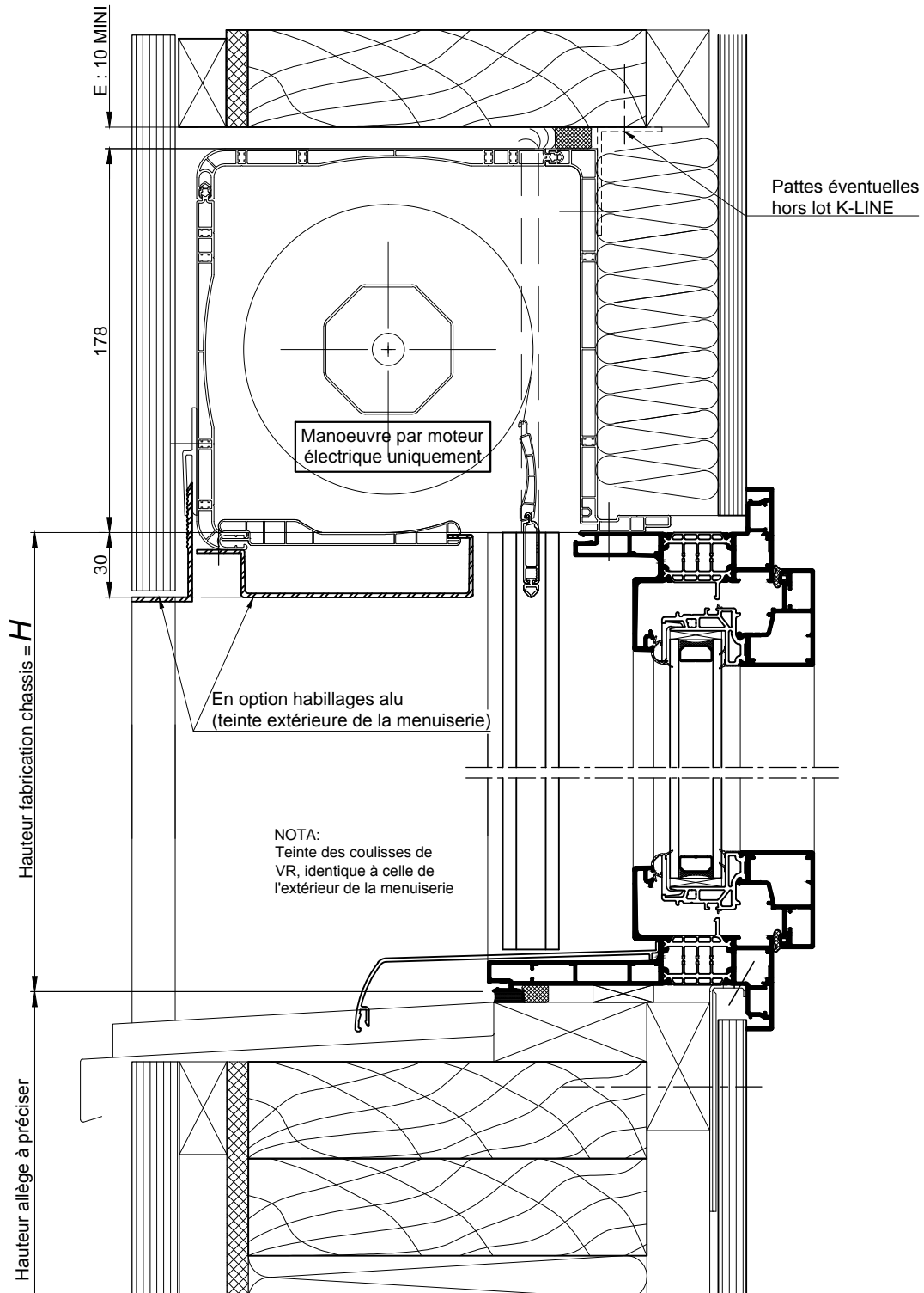
COUPE VERTICALE Ech 1/3
