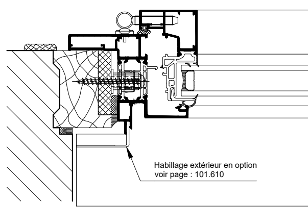
COUPE VERTICALE PARTIELLE Ech 1/3
