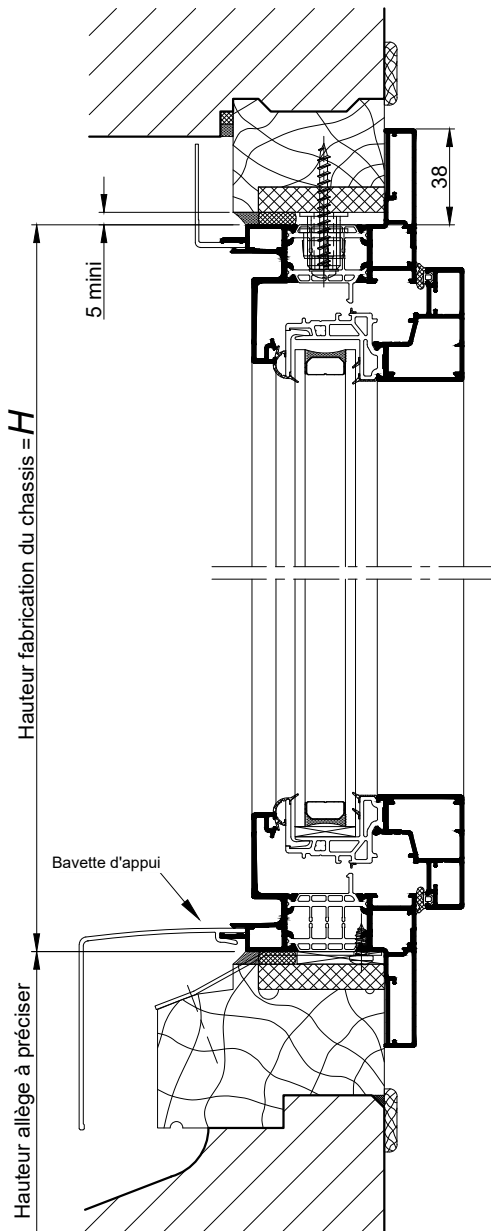
COUPE VERTICALE Ech 1/3
